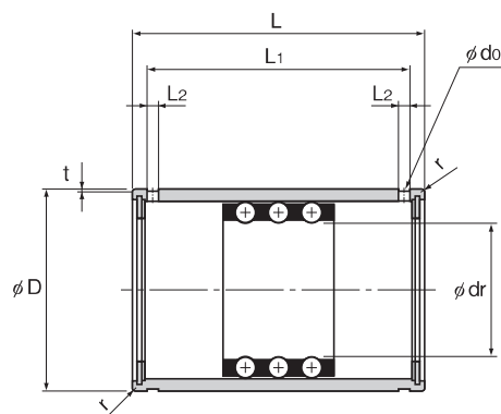
ST形 (軽荷重用)
