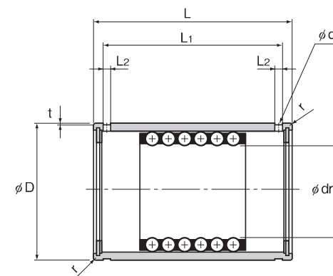
ST-B形 (中荷重用)
