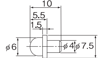
PB1021B形
