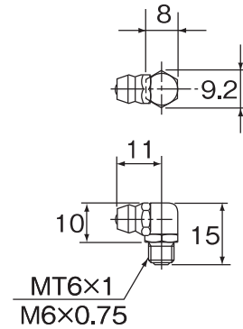
C-MT6×1形 (MT6×1) C-M6F形 (M6×0.75)
