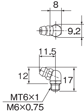
B-MT6×1形 (MT6×1) B-M6F形 (M6×0.75)
