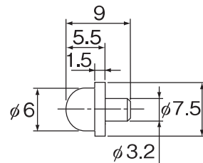
NP3.2×3.5形
