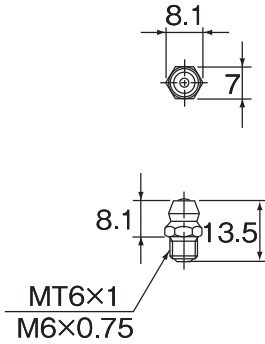
A-MT6×1形 (MT6×1) A-M6F形 (M6×0.75)
