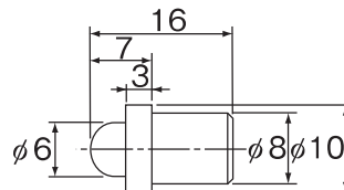
NP8×9形
